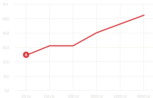
A SpaceM Schalldämmung [dB] x - Frequenz [Hz] y - Schalldämmung [dB]
